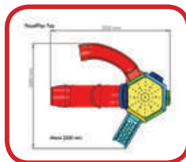
31222 - C : Royal Play Top (c/ 1 escorregador + esca- lada + tubo) Idade: Até 12 anos Alt.: 1,85 m Larg.: 3,25 m Profundidade: 2,65 m
